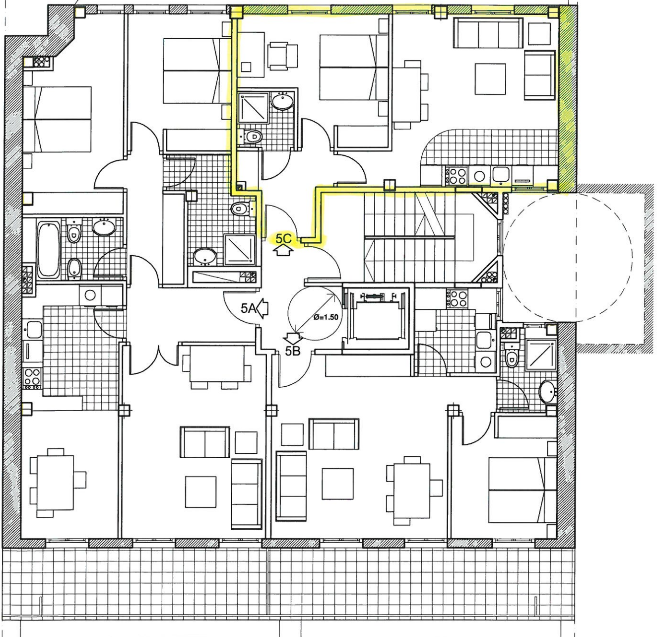
PLANTA QUINTA
